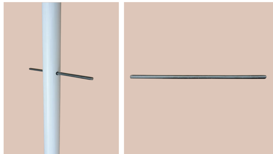
ネカセ棒 (回転・引き抜き防止) \phi 9 \times 300
