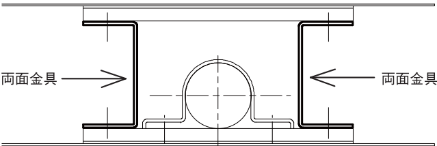
コの字金具取付参考平面図
