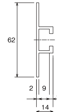
平リブ断面図
