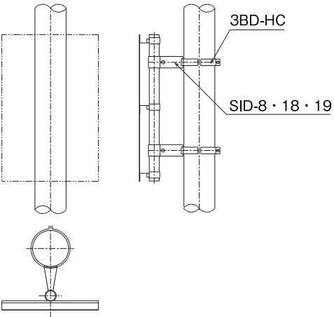
コンクリート柱設置参考図
