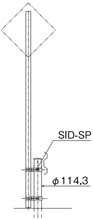
ガードレール共架設置参考図
