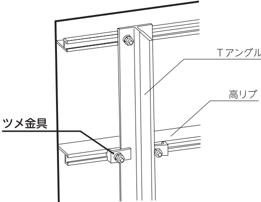
ツメ金具取付参考図
